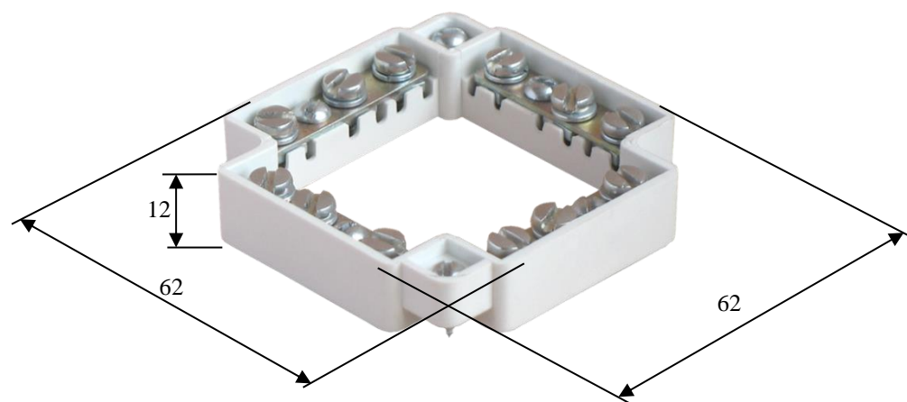
Рисунок 1 Габаритные размеры
